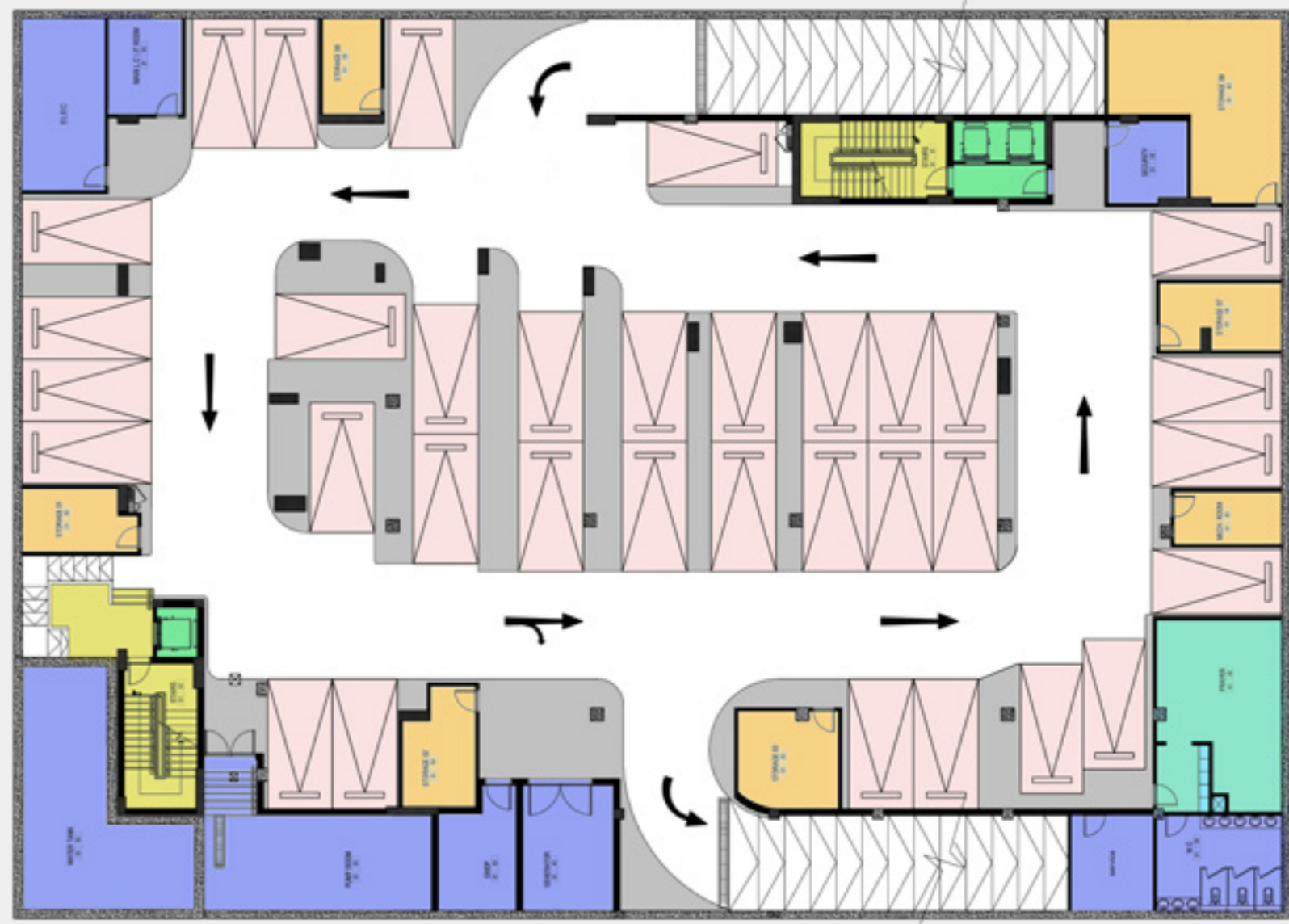
الطابق السفلي ■ خدمات ■ مصاعد ■ مخازن ■ مواقف سيارات ■ مكاتب ■ سلام
