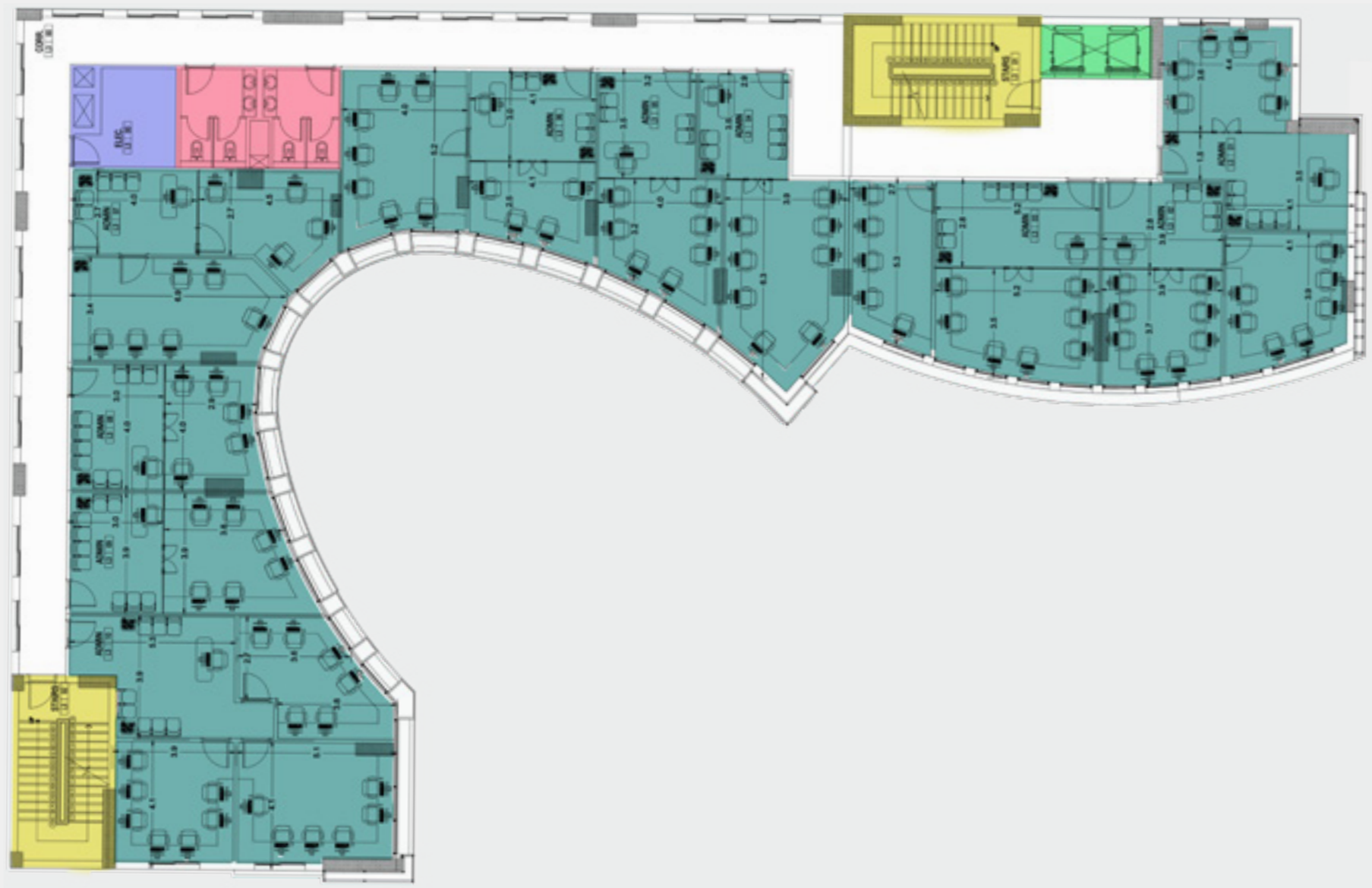
الطابق الثاني ■ خدمات ■ حمامات ■ مصاعد ■ سلام ■ مكاتب
